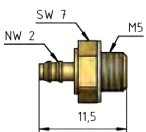
Threated Sleeve (incl. 1 seal) AV M5/3
